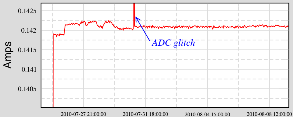
SLED Actual Current Delivered
