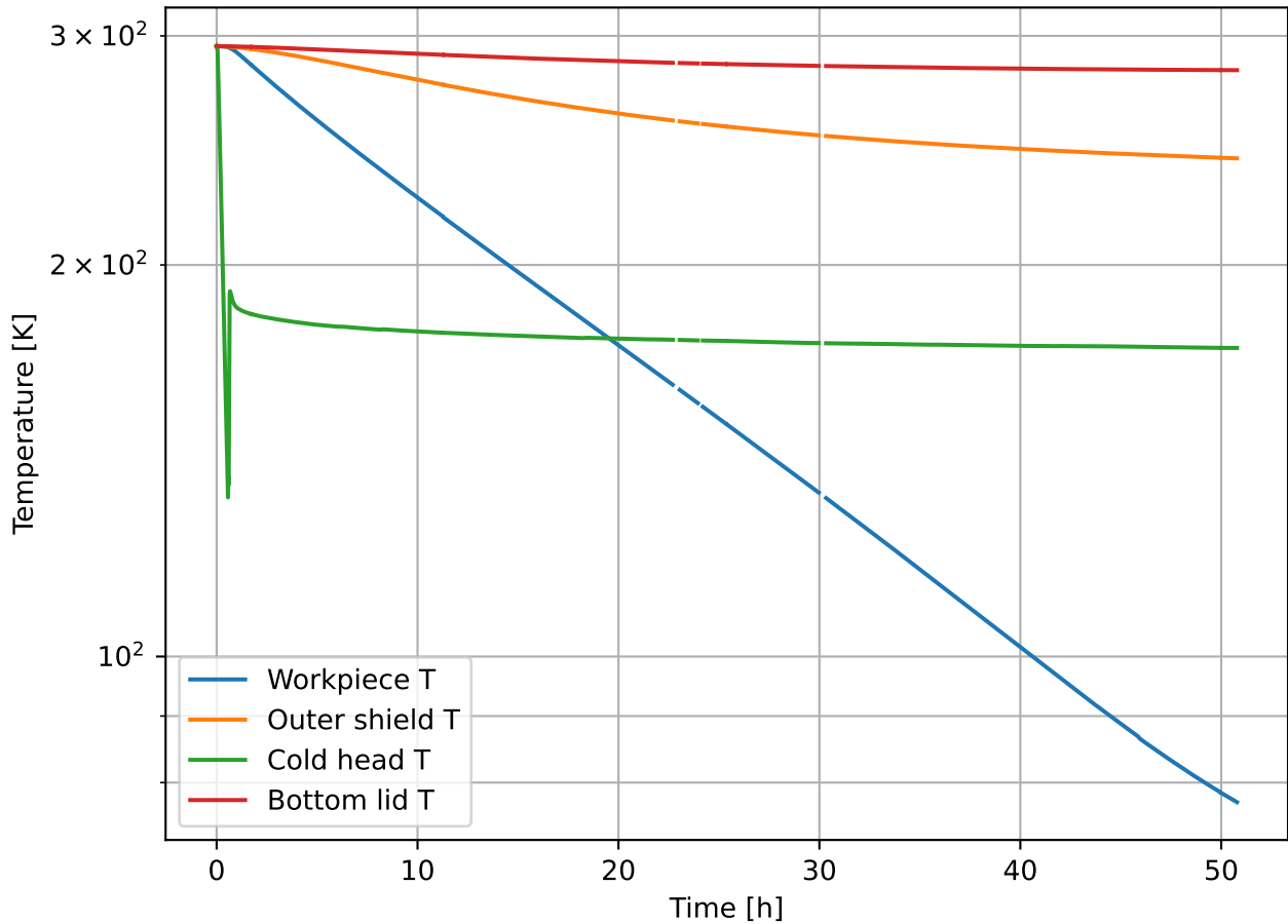
Cryochamber cooldown 6/21-6/24
