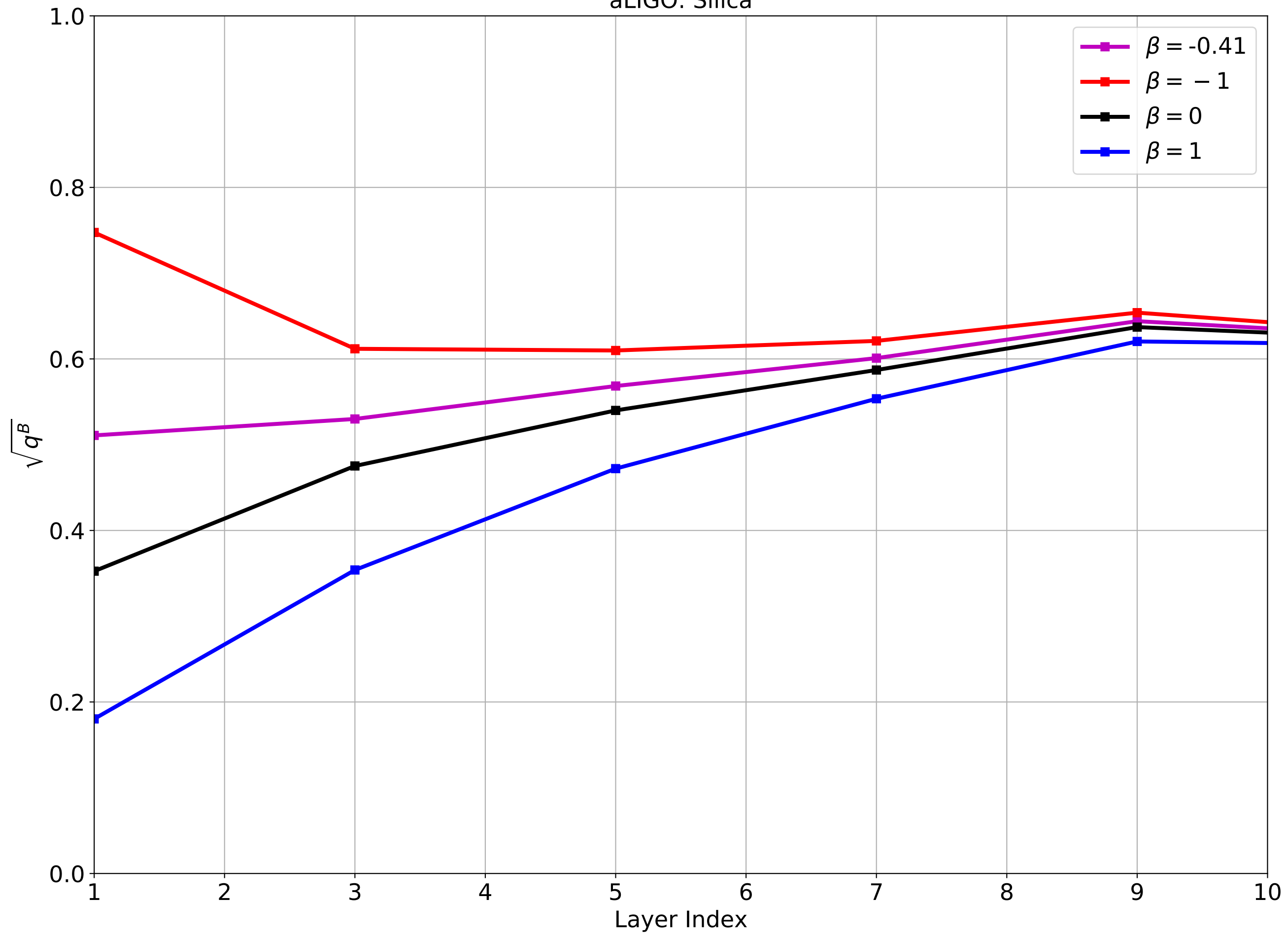
aLIGO: Silica
