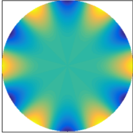
Mode 6, 6739.5 Hz
