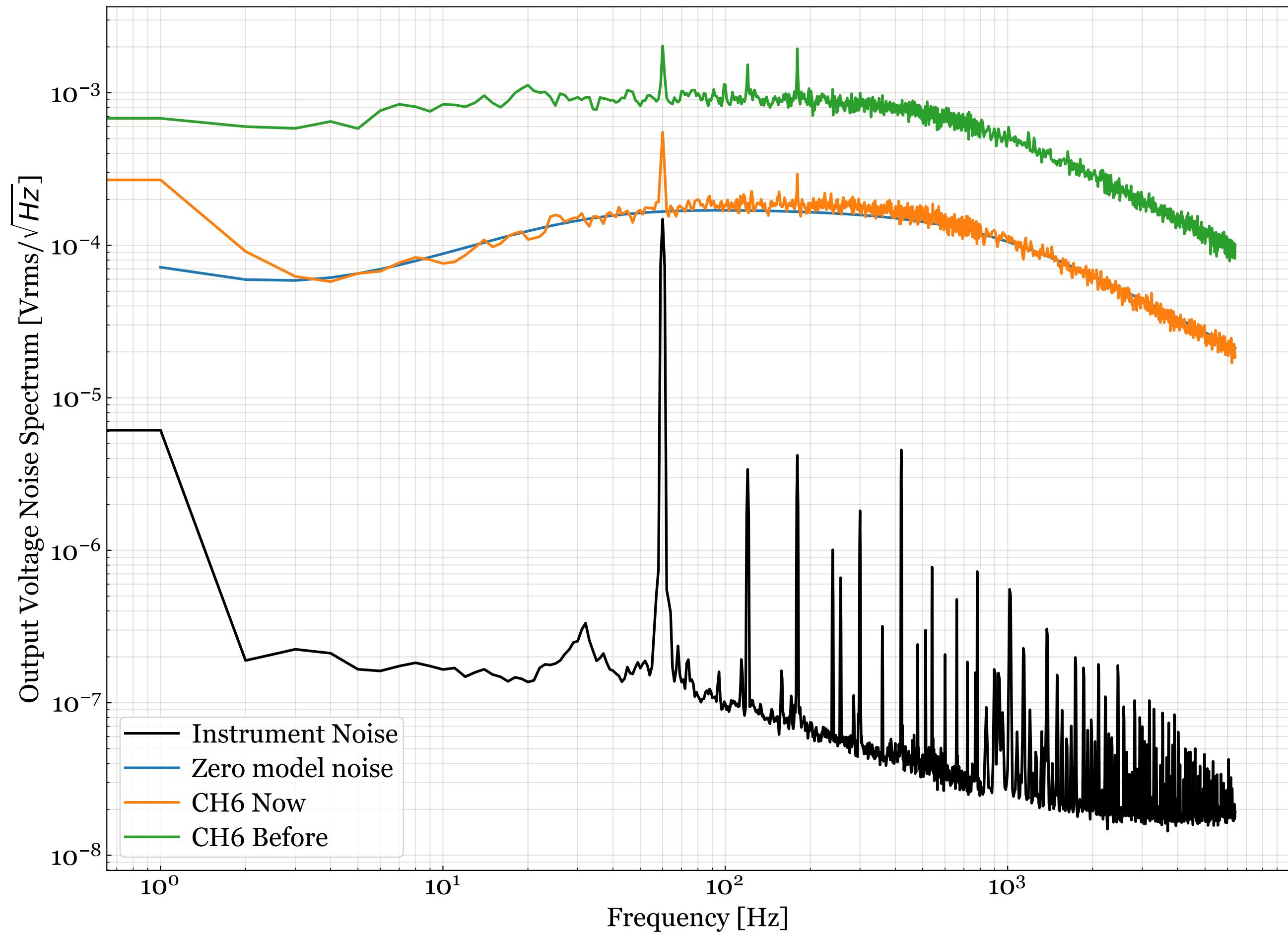
D11000687 S2100029 Output Voltage Noise Spectrum.
