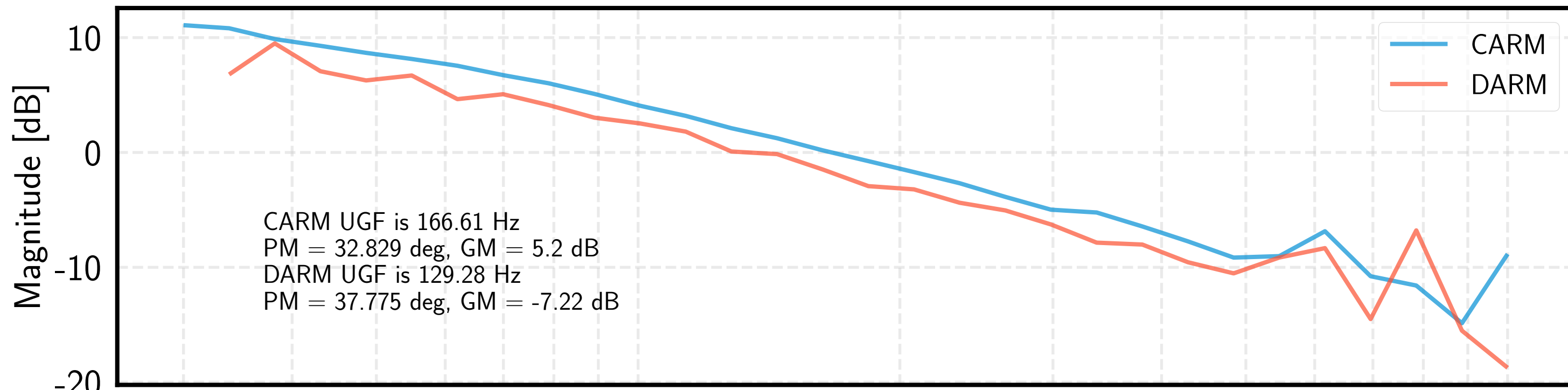
ALS CARM/DARM OLFs with CARM actuation on ETMs
