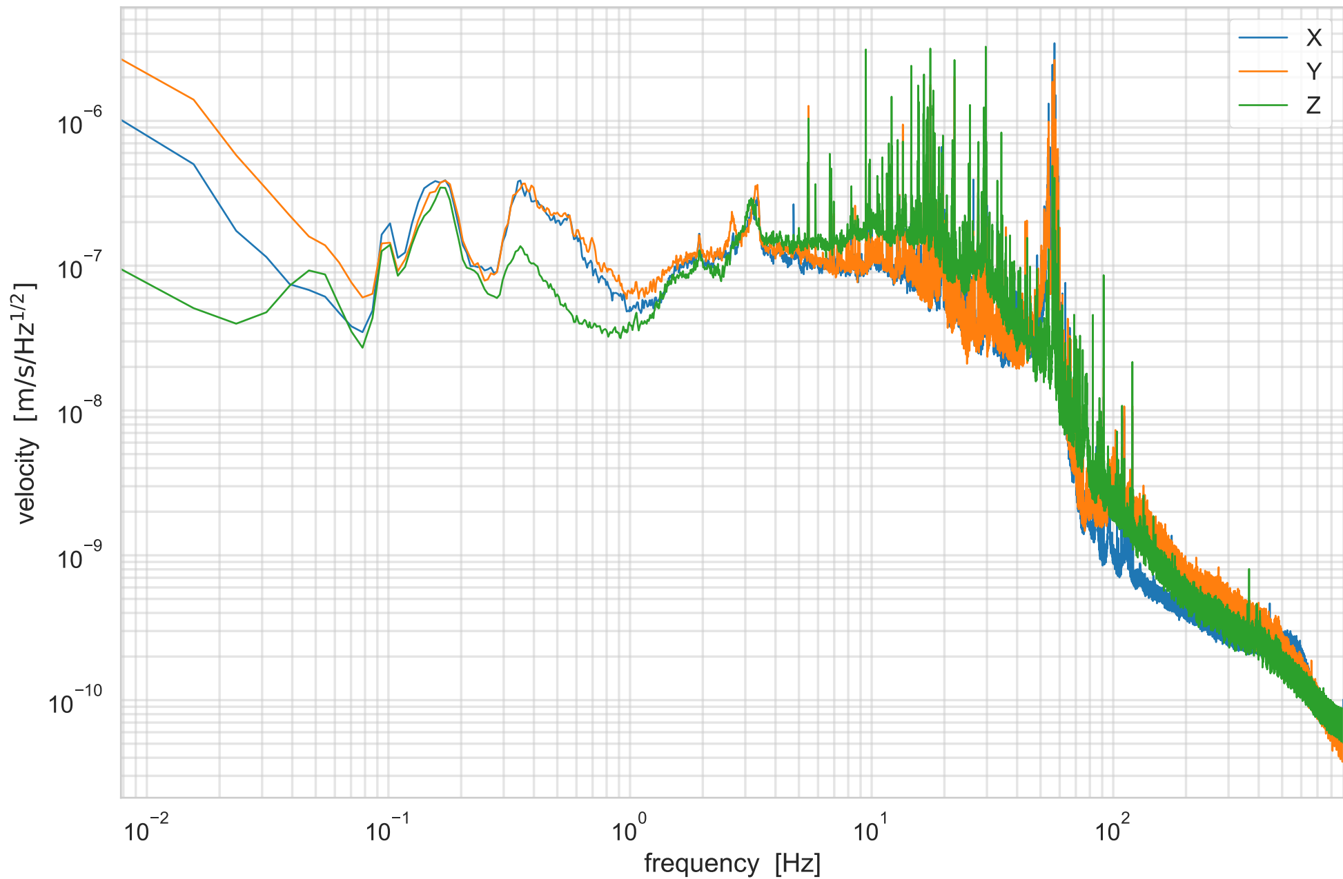
BS Trillium Seismometer Noise
