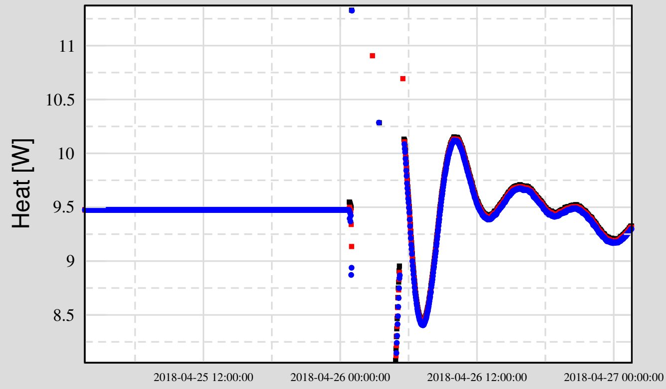
Ch 1: C1:PEM-SEIS_EX_TEMP_CTRL_WATTS
