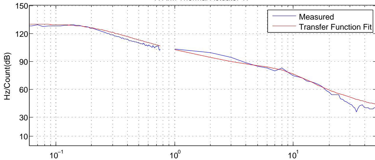
X Arm Thermal Actuator TF
