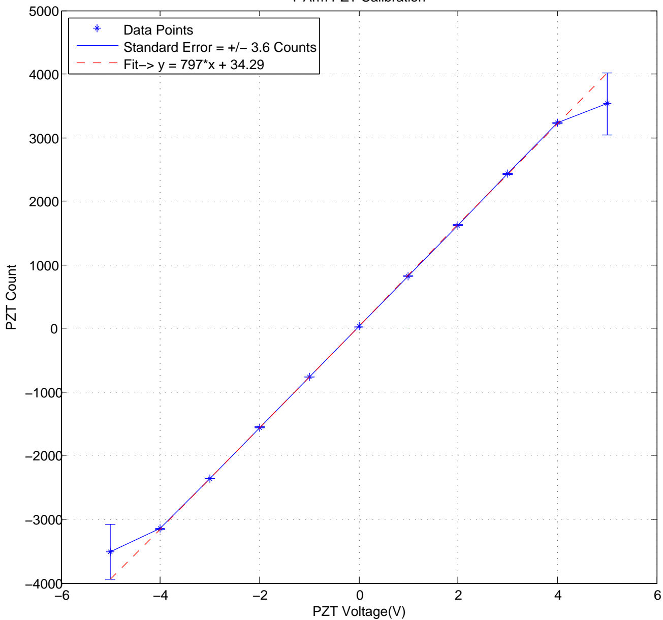
Y Arm PZT Calibration
