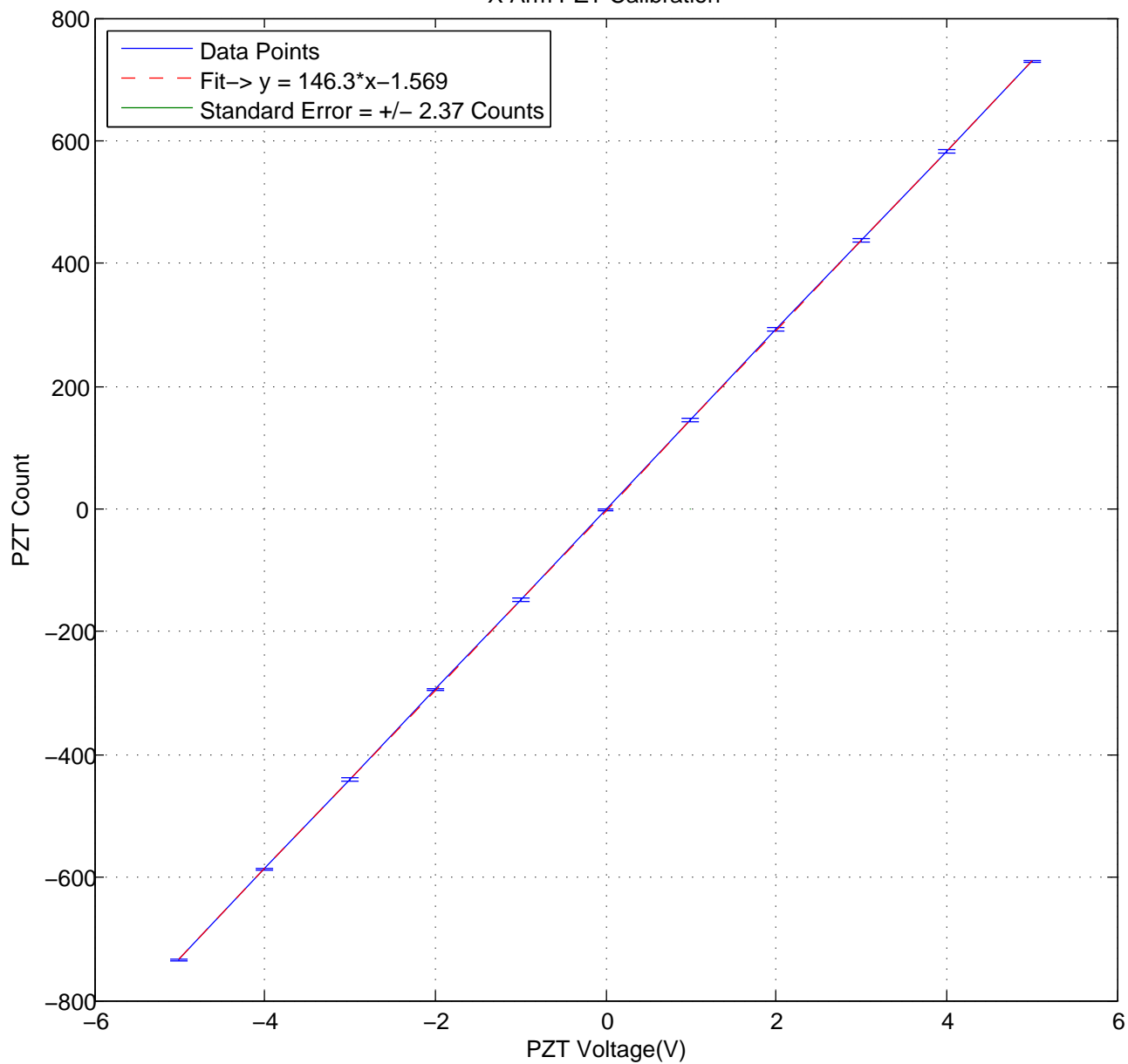
X Arm PZT Calibration
