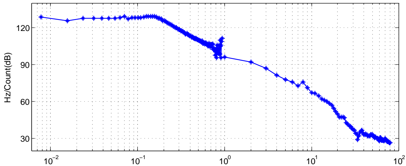
X Arm Thermal Actuator TF
