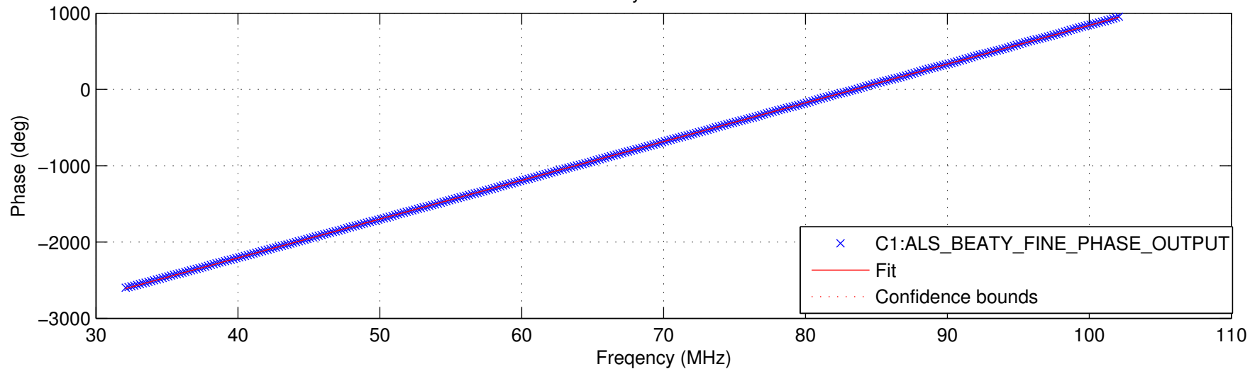
y vs. x1
