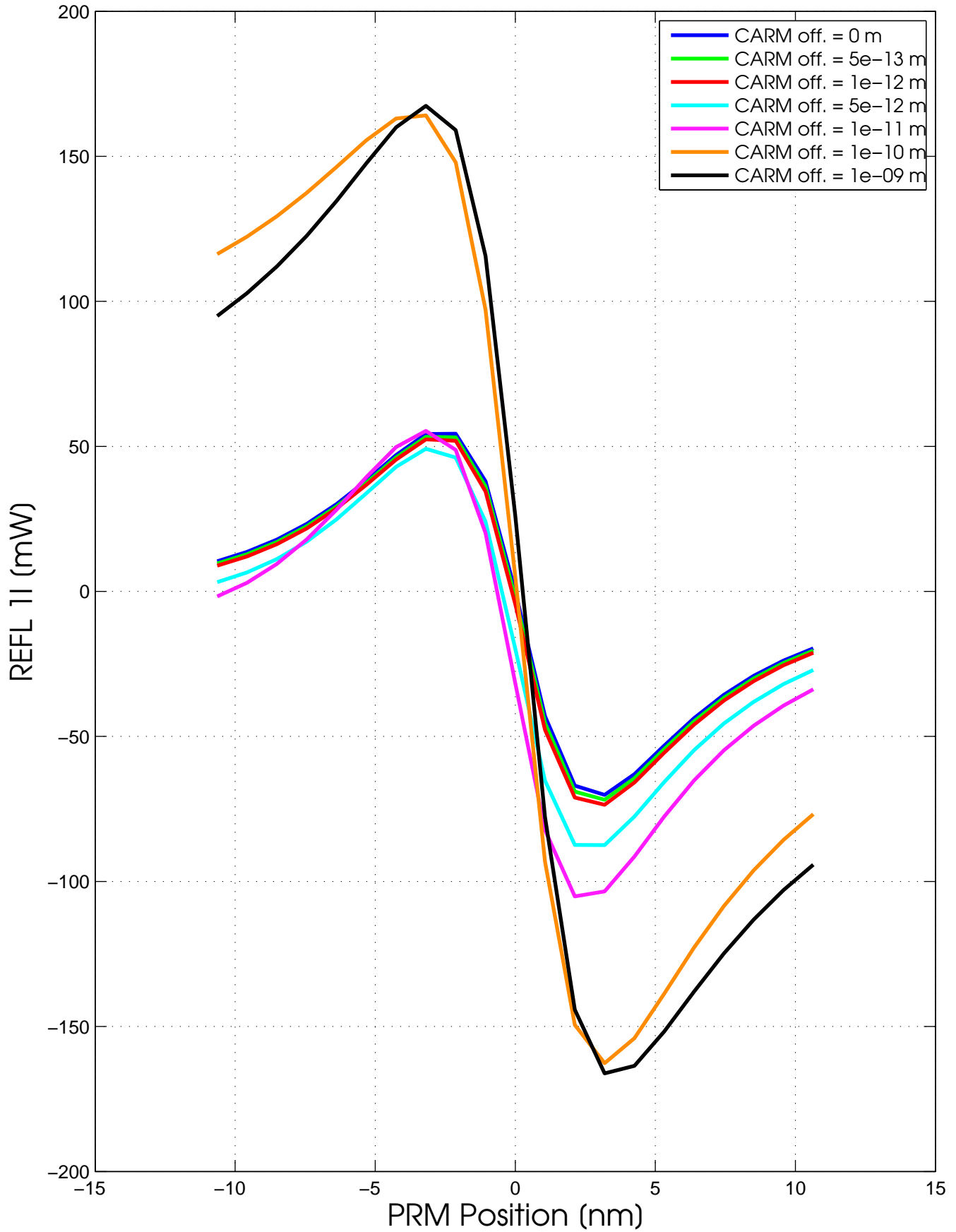
Current 40m PRCL f1 Demod I Phase
