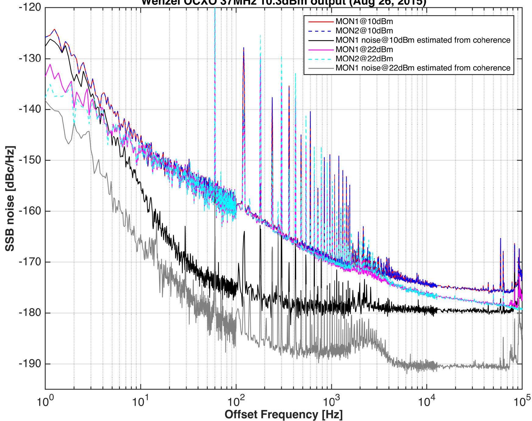
Wenzel OCXO 37MHz 10.3dBm output (Aug 26, 2015)
