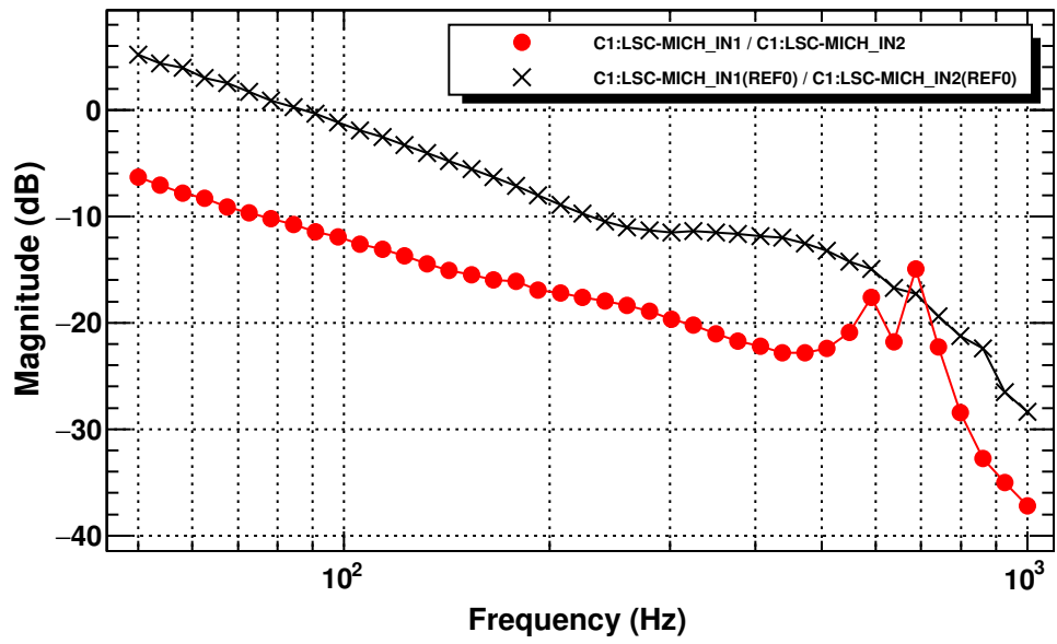
MICH Open Loop Gain
