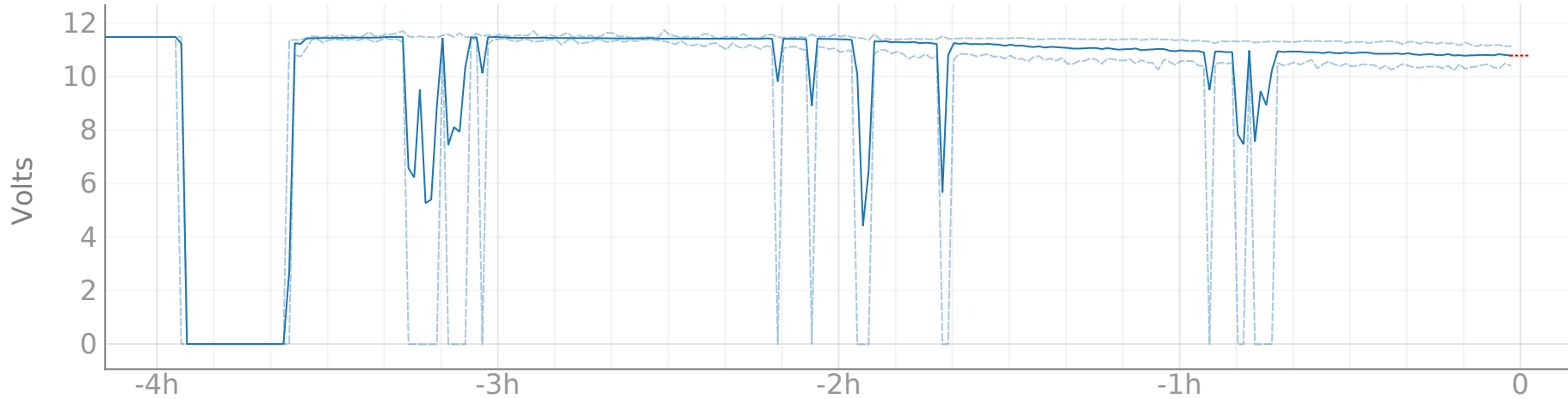
C1:ASC-IP_POS_QPD_X_Calc [m-trend]
