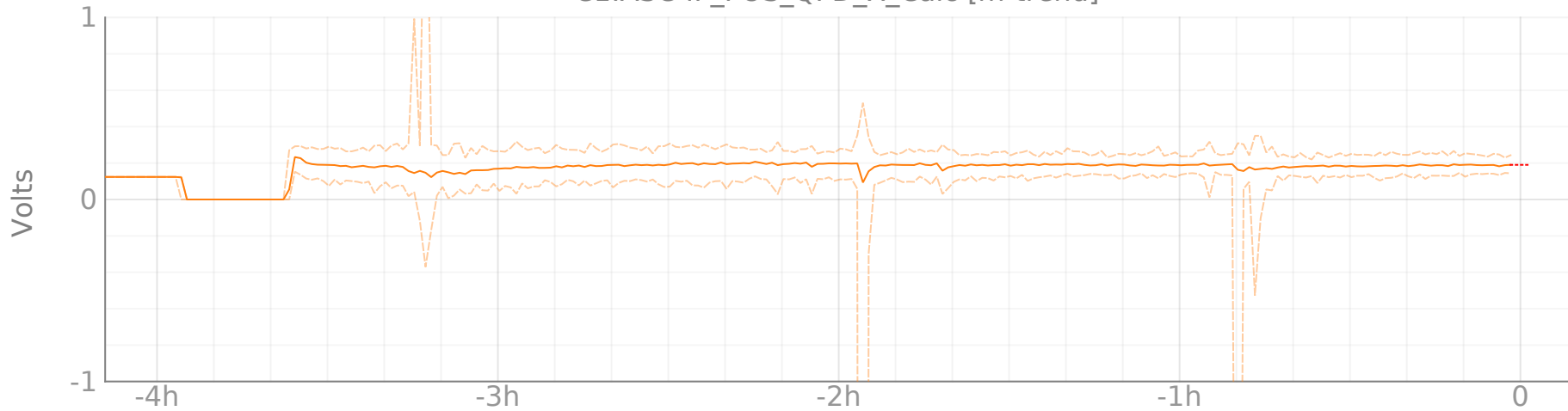
C1:ASC-IP_POS_QPD_Y_Calc [m-trend]
