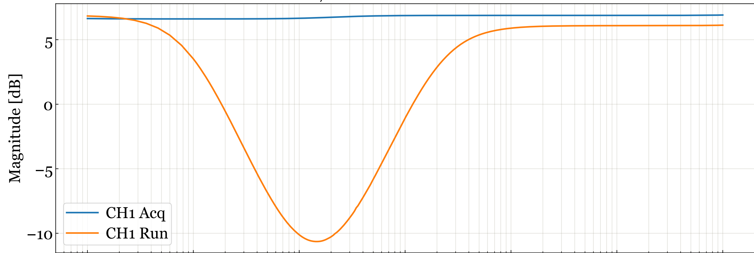
D11000687 S2100028 CH1 Transfer Function
