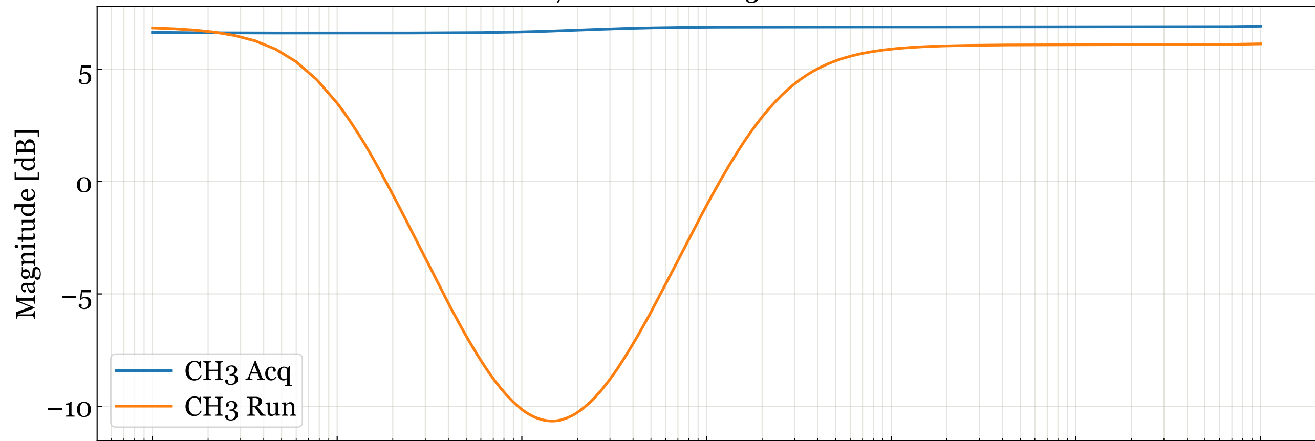
D11000687 S2100028 CH3 Transfer Function
