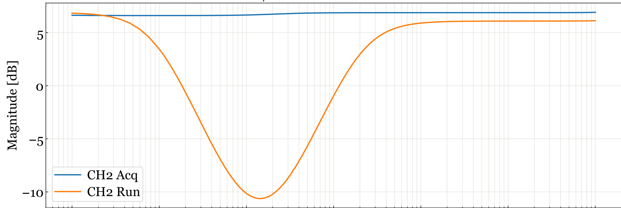
D11000687 S2100028 CH2 Transfer Function
