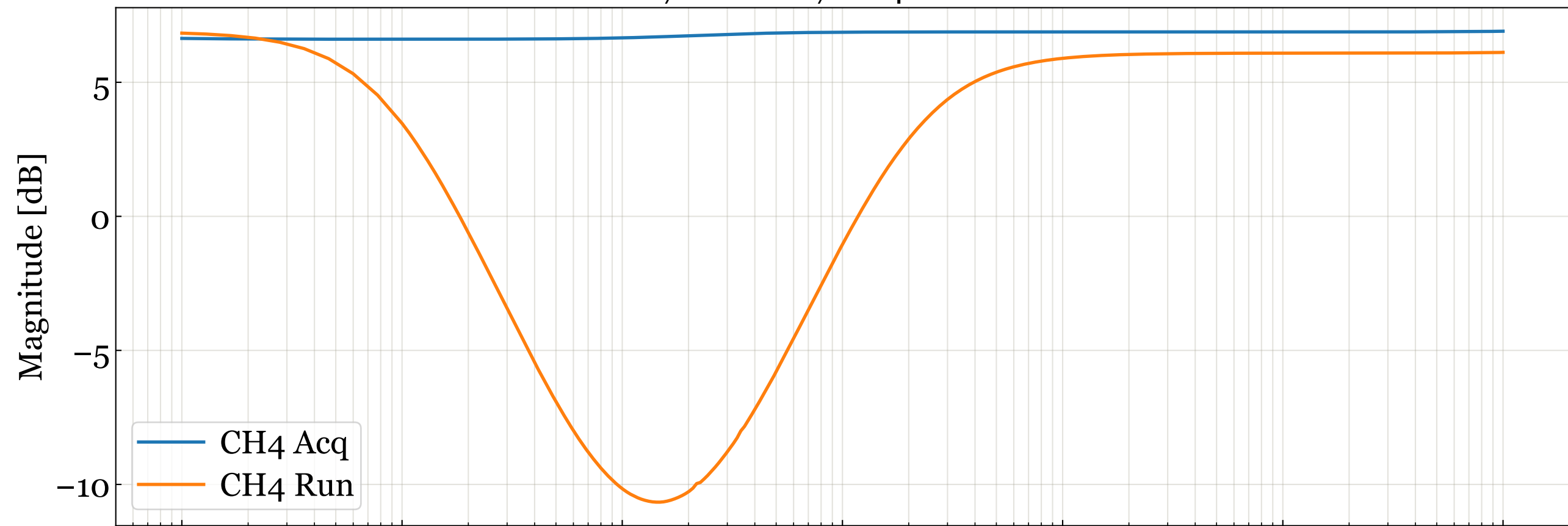
D11000687 S2100027 CH 4 Transfer Function
