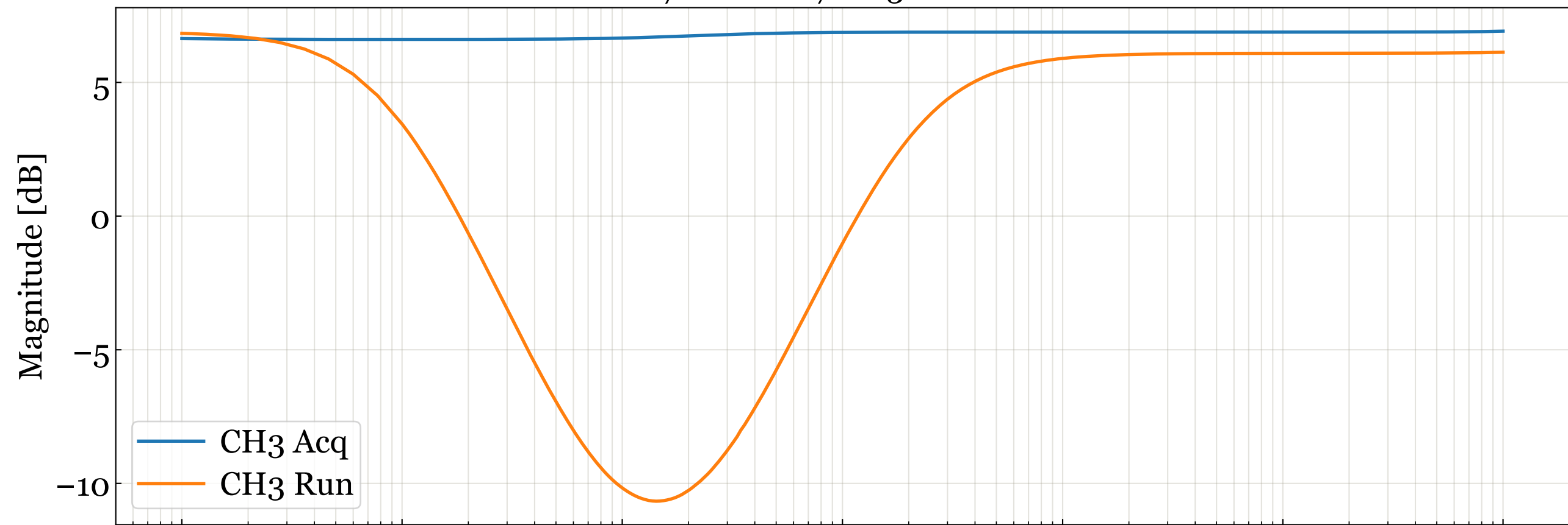
D11000687 S2100027 CH3 Transfer Function
