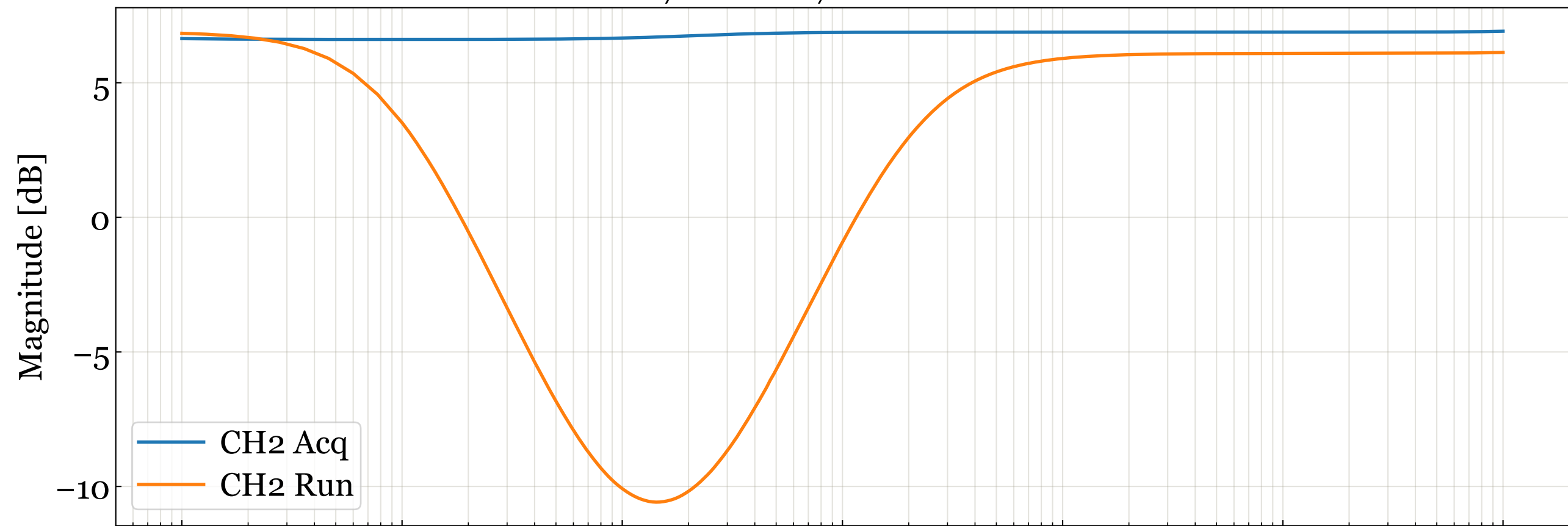
D11000687 S2100027 CH2 Transfer Function
