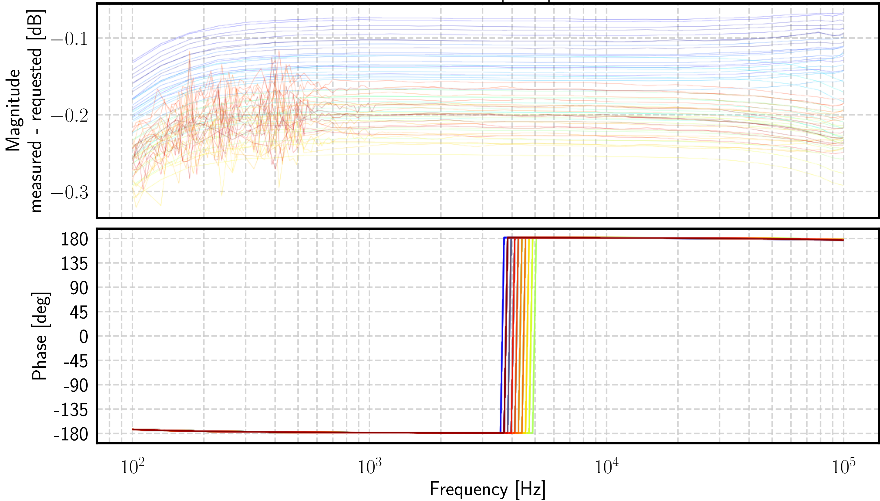
IMC Servo board AO path input TFs
