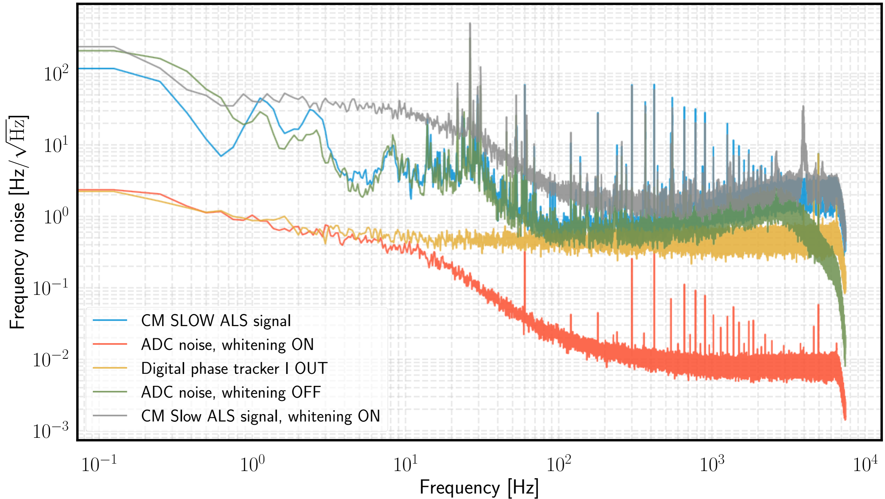
Testing the CM SLOW ALS (X) signal path
