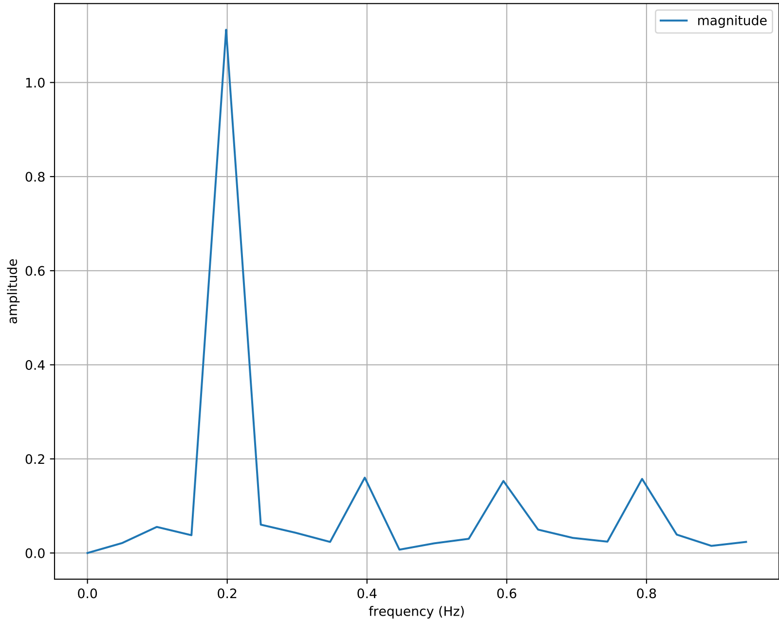
FFT_yaw
