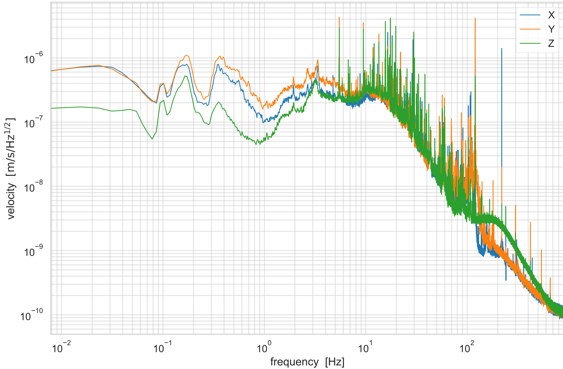
EY Guralp Seismometer Noise
