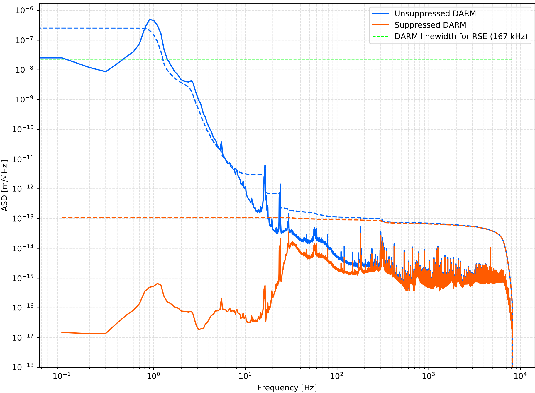
DARM loop suppression for assumed OLG
