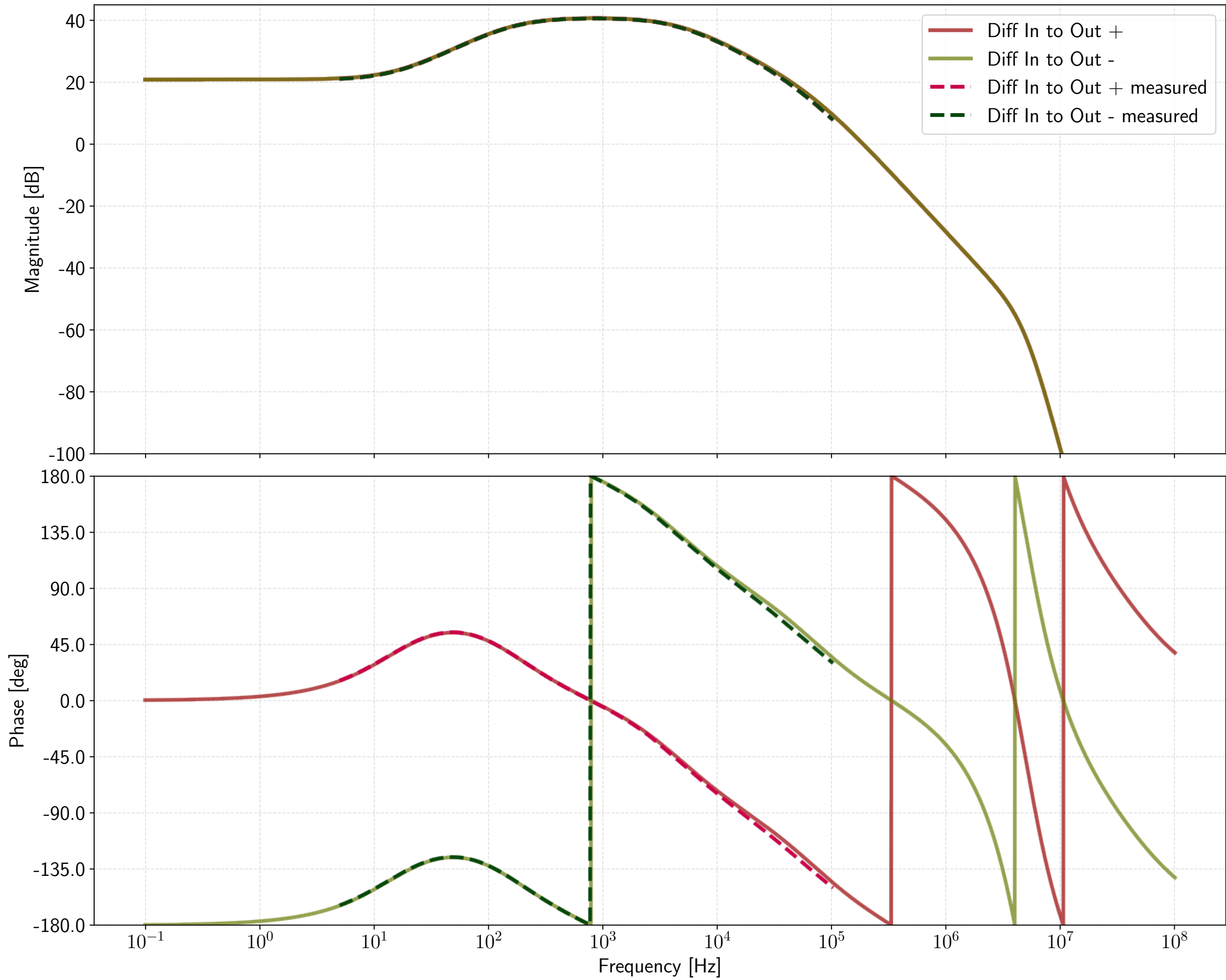
ALS proposed IF amplifier/whitening daughter board TF
