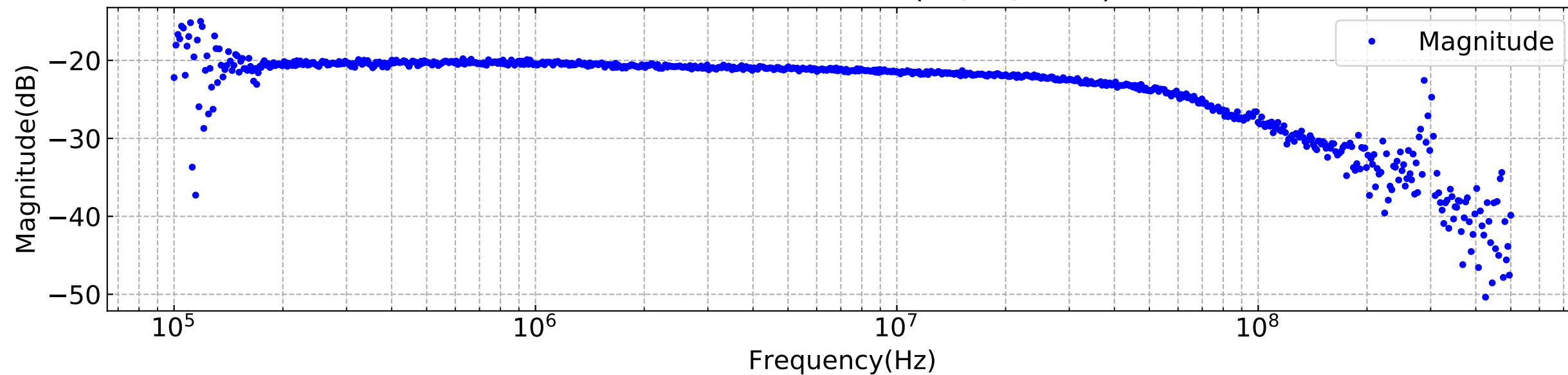
LIGO ET-3040 PD Test(19/05/2017)
