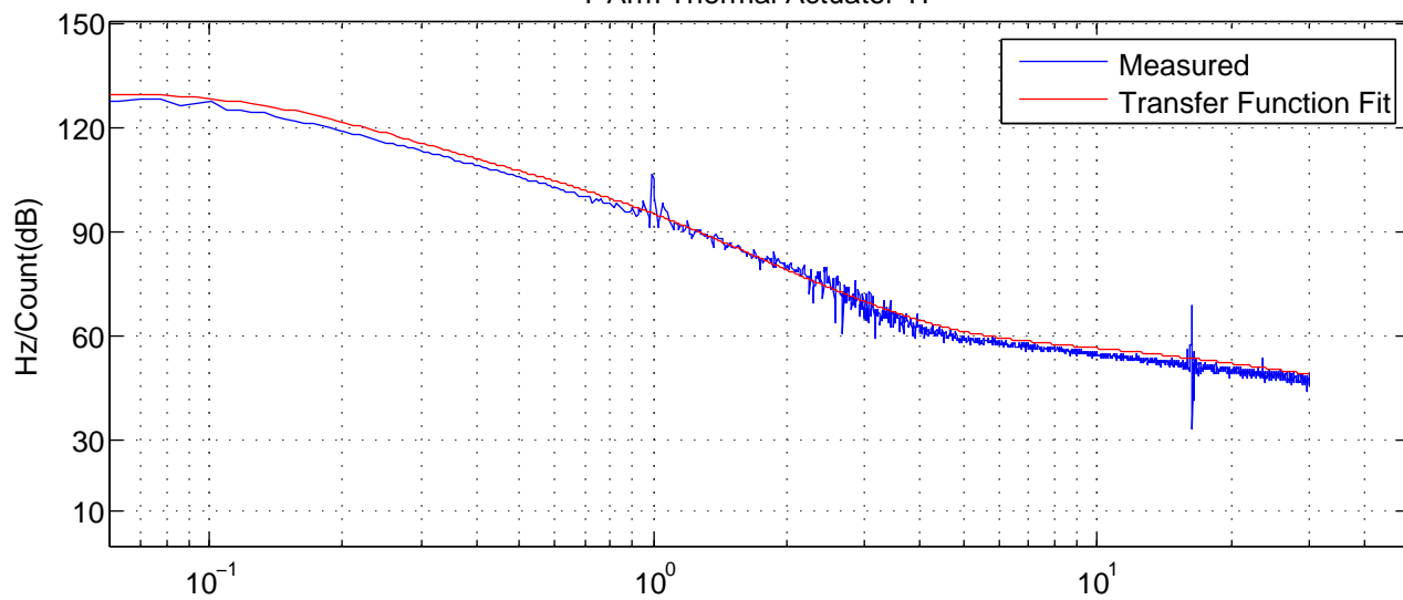
Y Arm Thermal Actuator TF
