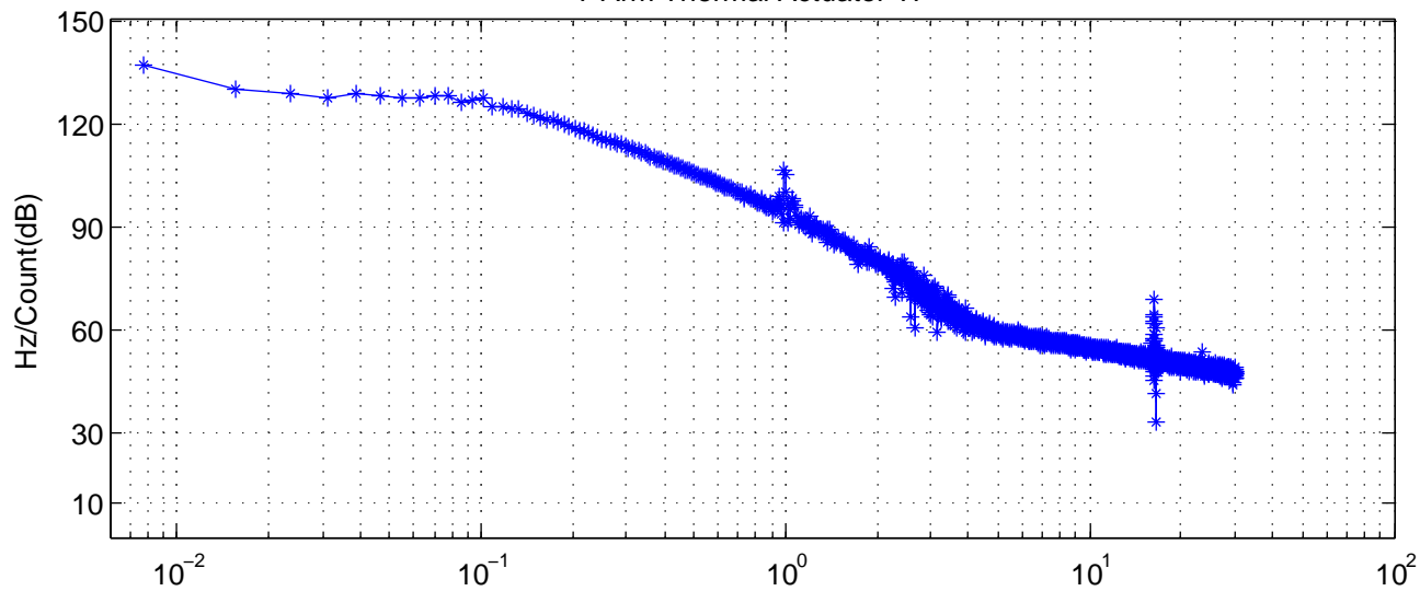
Y Arm Thermal Actuator TF
