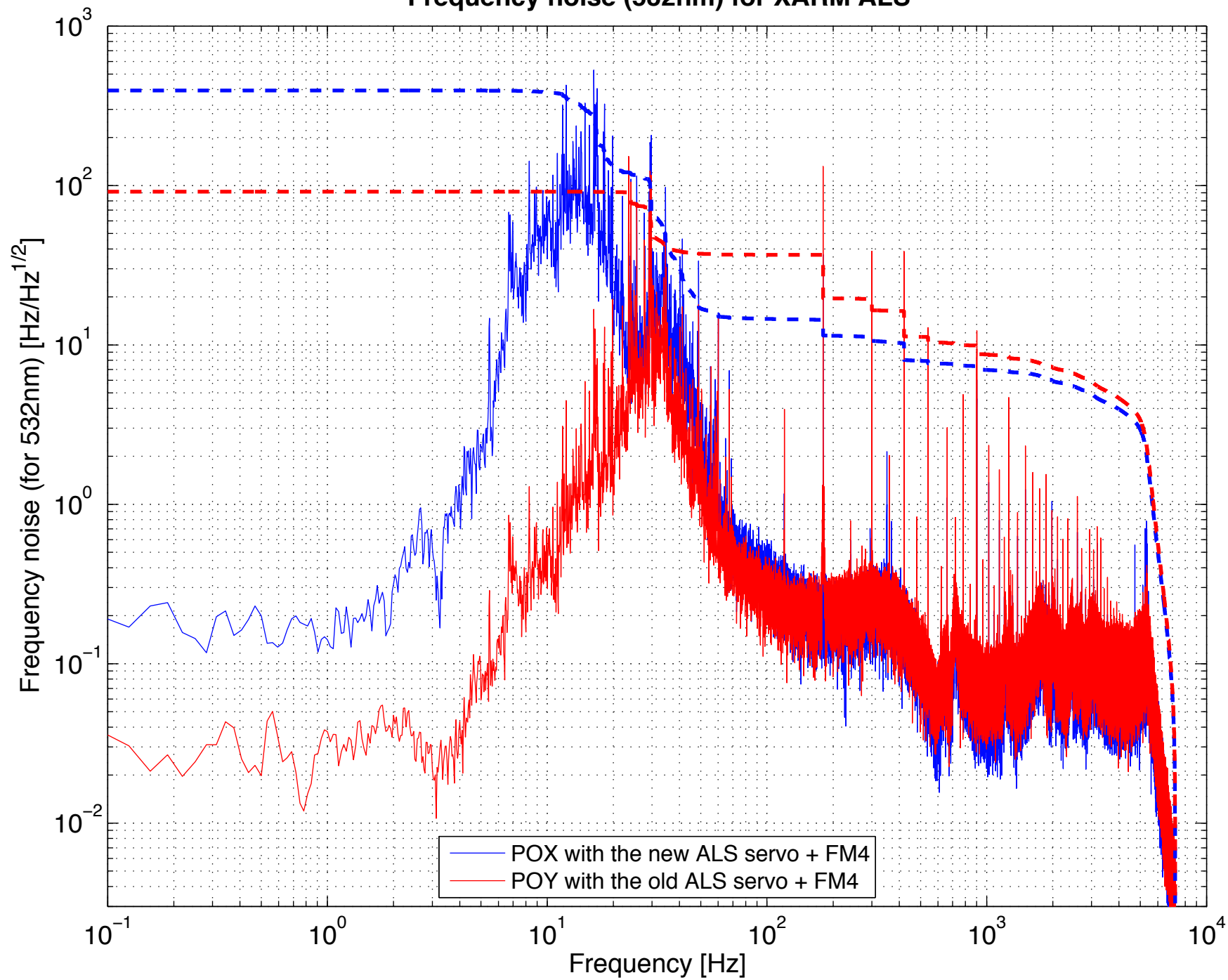
Frequency noise (532nm) for XARM ALS
