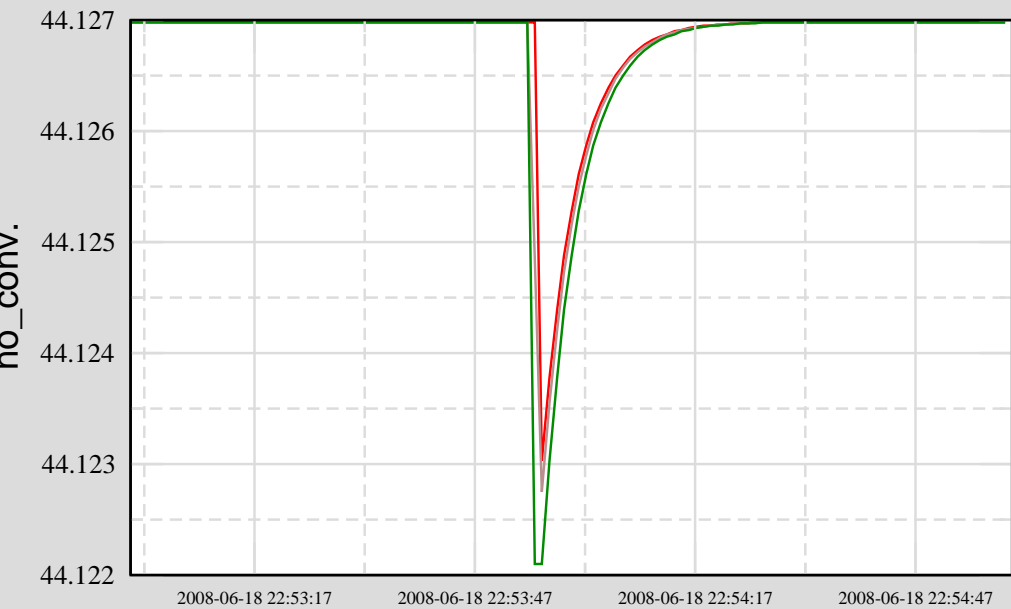
Ch 3: C1:PSL-126MOPA_LTMP
